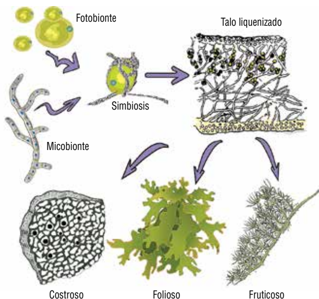
Figura 1: Formación de un líquen y tipos (Dibujo original: C. Maldonado, P. Rodríguez). 1
