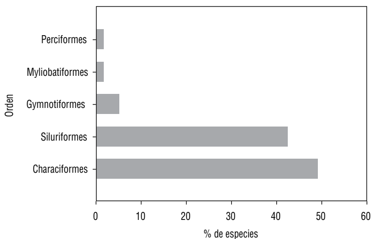
Figura 2. Composición por órdenes de peces registrados en Sara Ana y sus alrededores.
