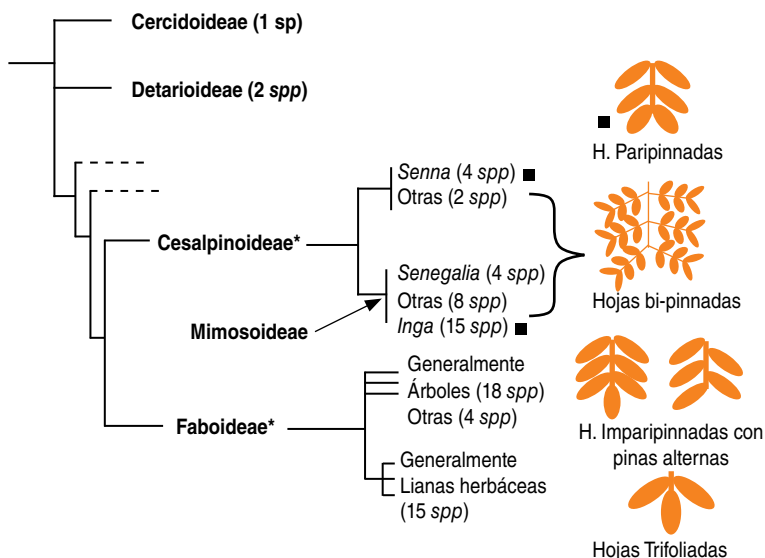
Figura 1: Esquema de la diversidad de leguminosas presente en Sara Ana, relaciones filogenéticas y algunos patrones morfológicos. Elaboración propia. *hace referencia a que se trata de Caesalpinoideae sensu stricto en base a la propuesta de LPWG 2017.
