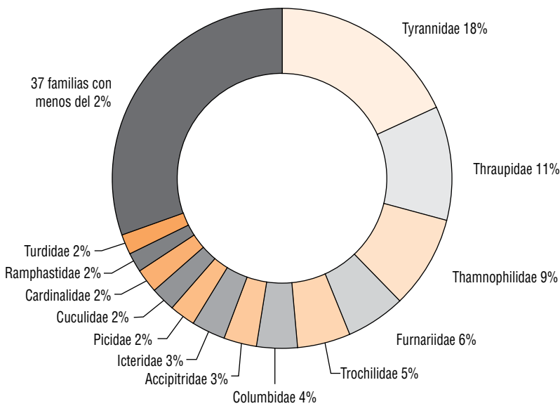
Figura 1: Porcentaje de especies por familia registrada en Sara Ana y sus alrededores
